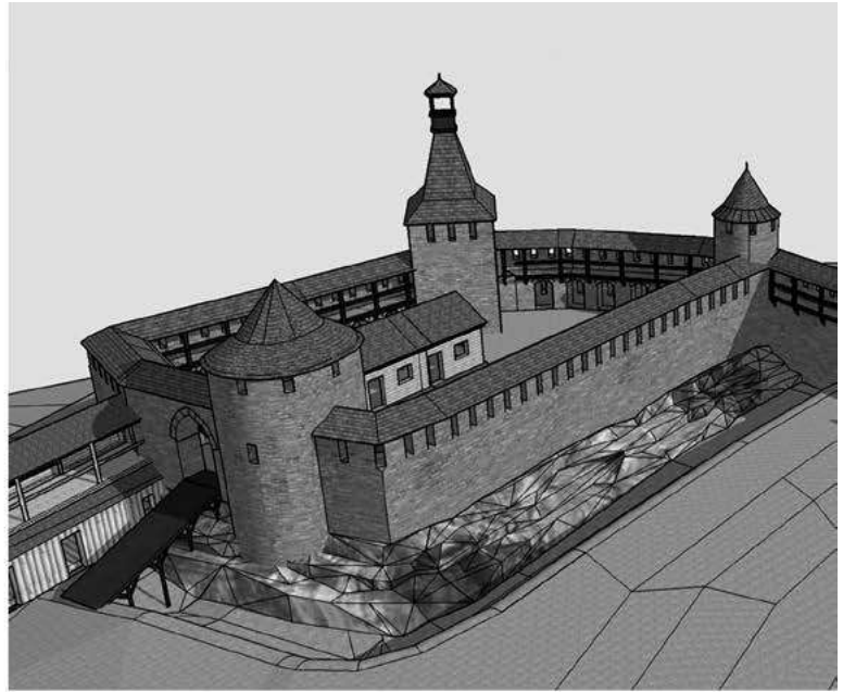
Рис. 2. Північна кам'яна частина замку, XII-XIII ст. Гіпотетична реконструкція. Автор 3D моделі – Бабюк Д.
