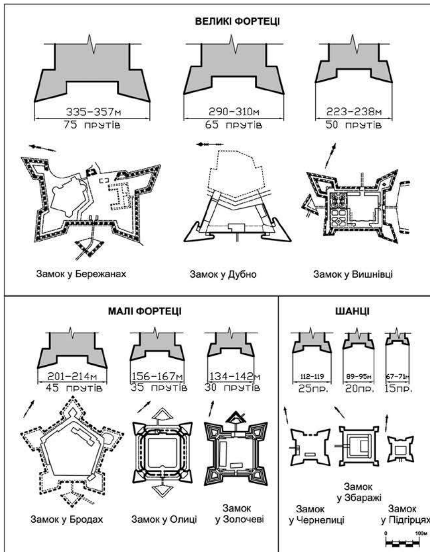
Рис. 2. Порівняльна схема абрисів бастионних замків Західної України, розподілених відповідно до класифікаційного поділу укріплень з трактату Й. Нароновіча-Нароньського.
