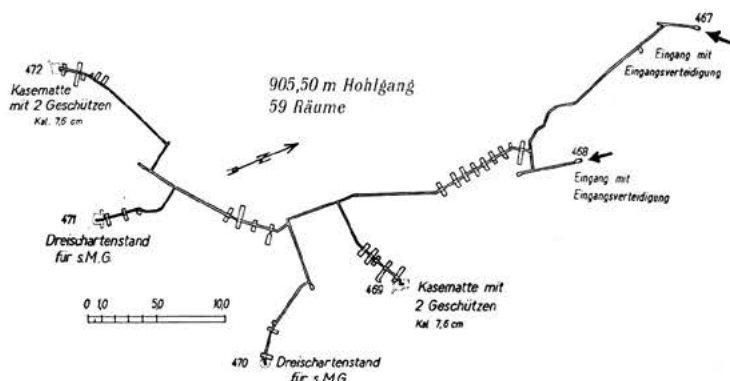
Рис. 1. Схема Серебрійської міни №86 а-г (Denkschrift über die russische Landesbefestigung. Berlin: Gedruckt in der Reichsdruckerei, 1942 )
