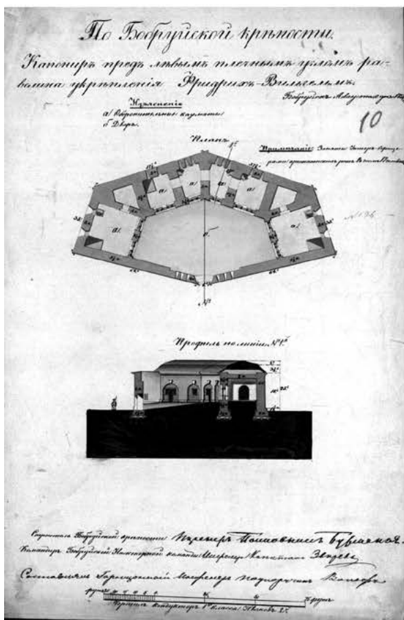
Рис.2. Капонира перед левым плечным углом рavelина укрепления Фридрих Вильгельм (НИАБ, ф.1477, оп.1, д.136, л. 10)
